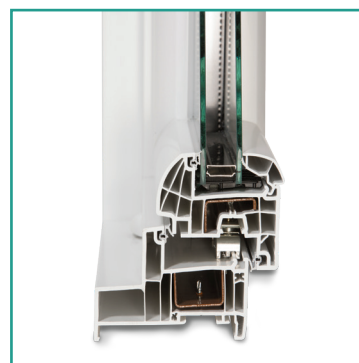
Coupe ouvrant/dormant 83 mm (6 chambres)
