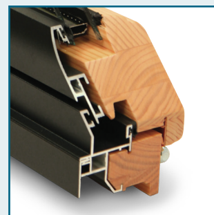
Double joint à frappe
