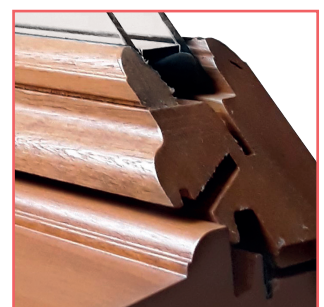
Drainage rapide Double joint à frappe
