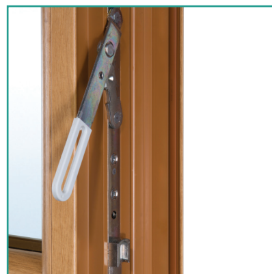
Verrou de sécurité sur semi-fixe
